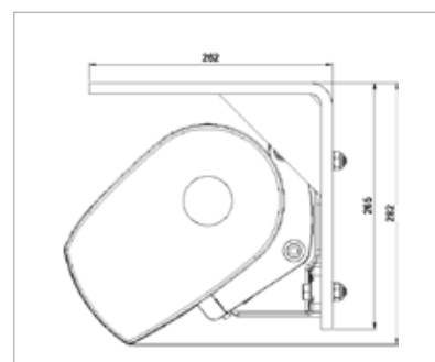
Fijación a techo - regulación máxima
