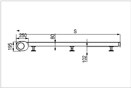
Vista lateral del producto
