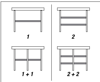
Posibles variaciones de tubos intermedios
