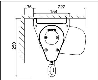
Instalación a techo Rail frontal redondeado
