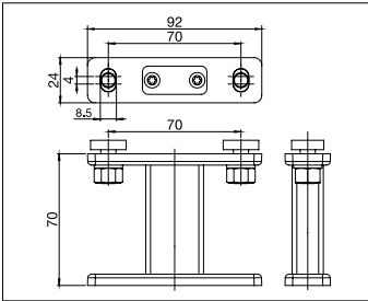
PS401/1 Soporte
