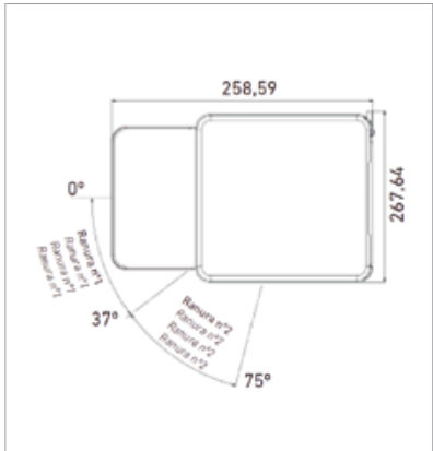
Dimensiones básicas
