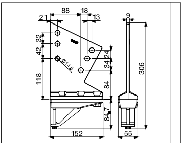
S825 Soportes pequeños techo/muro
