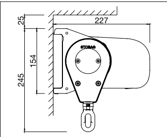
Instalación a pared Rail frontal redondeado
