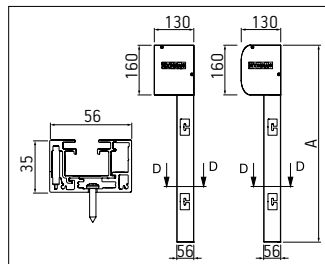
Montaje entre paredes A = Altura total
