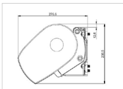
Fijación a muro - regulación máxima
