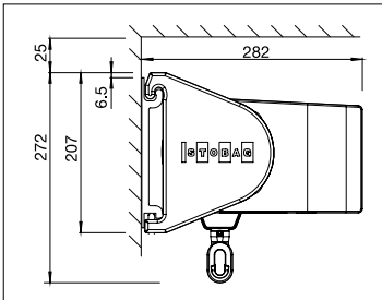
Vista lateral Instalación a pared - cuadrado
