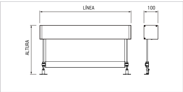
Dimensiones máximas del sistema con cable
