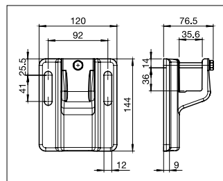
S221/1 Soporte para techo
