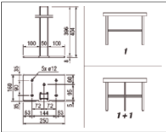
Placa base Variante de rodillos
