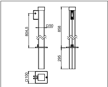
SR414/2 Kit poste para empotrar
