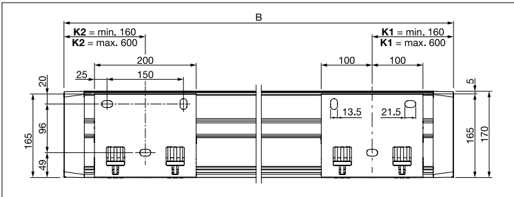
Plano de montaje (montaje a muro)
