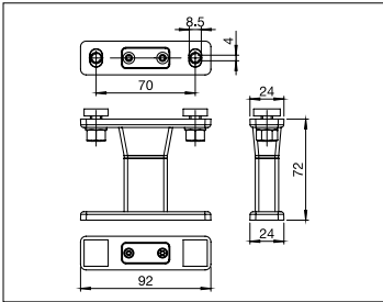
PS401/8 Soporte de fijación con Silent Block
