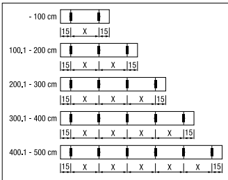
Disposición y número de soportes de montaje / punzones o clips
