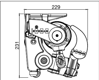
S8135 Instalación entre muros
