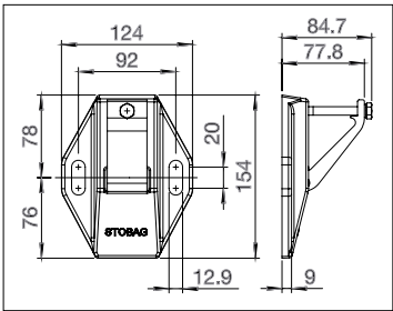
S821/1 Soportes techo/muro
