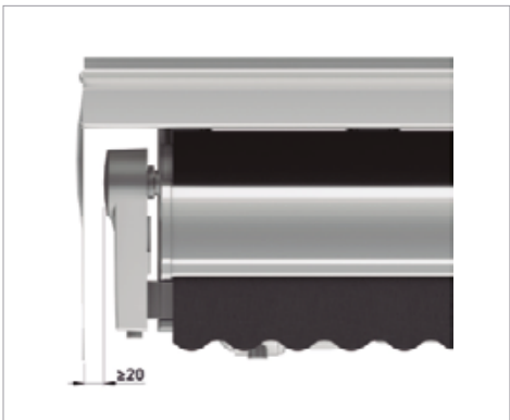
Espacio mínimo recomendado entre las tapas del tejadillo y los soportes.
