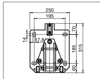
S340 Pie de la base S341 Soportes intermedios pared/techo
