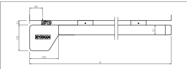
Largo total
