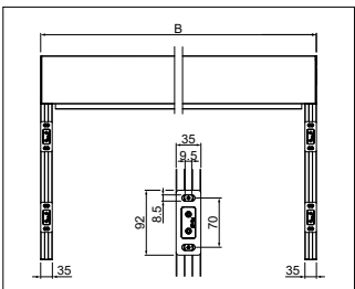
Disposición de los soportes con sistema de clips B = Anchura total
