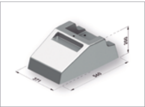
Lastre de hormigón
