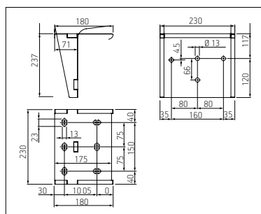
Herraje para montaje a techo
