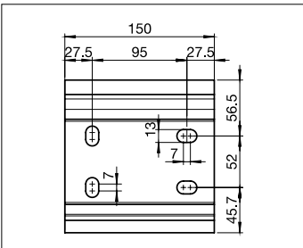
S721/2 Perfil de soporte L = 150
