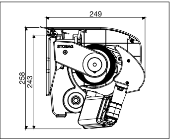
S8130/2 Instalación a pared con tejadillo S877/2
