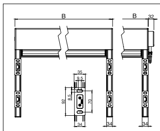
Disposición de los soportes con soportes B = Ancho total
