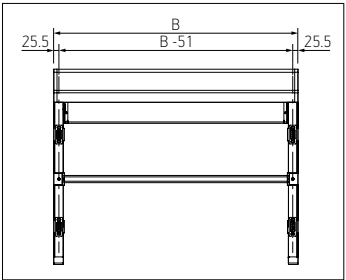
Plano de montaje B = largo total
