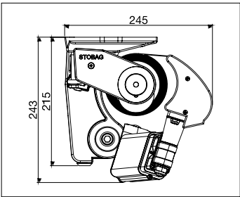
Instalación entre paredes
