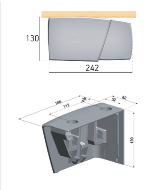
Fijación a techo
