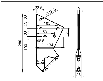
S825/1 Soportes para viga (vista frontal)
