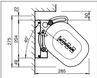
Instalación a pared 40°
