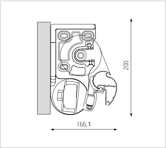
Montaje a pared
