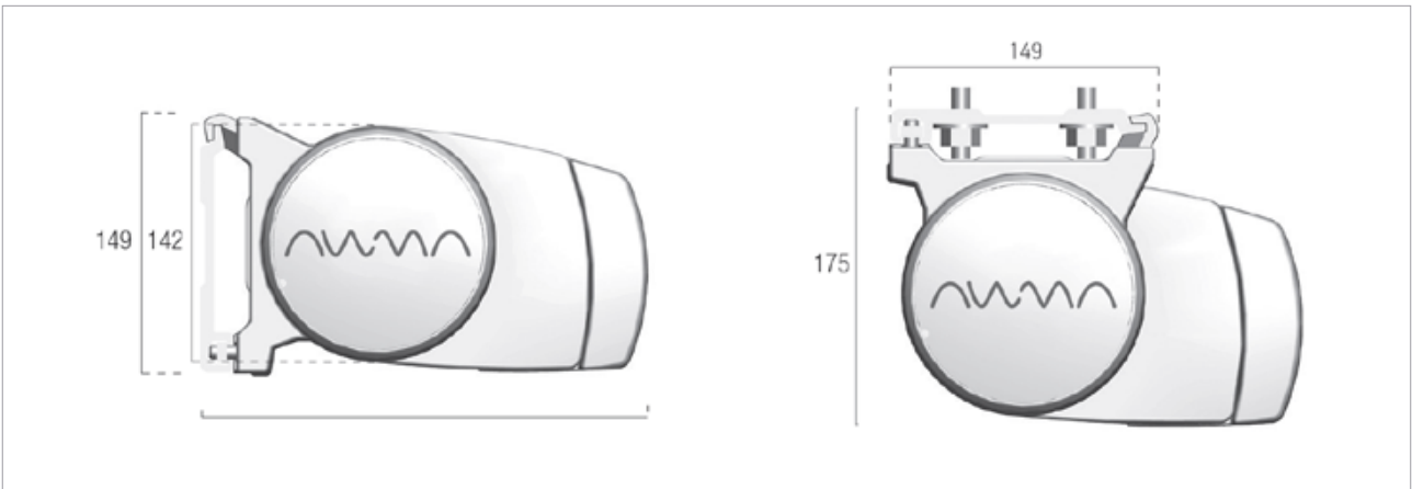
Instalación frontal
