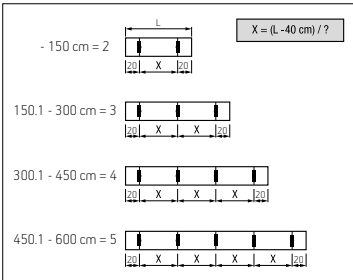
Reparto y nº de soportes sin ZIP
