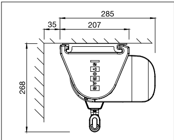
Vista lateral Instalación a techo - redondeado
