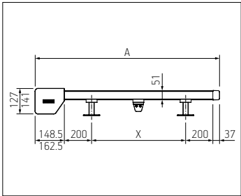
Vista lateral A = salida
