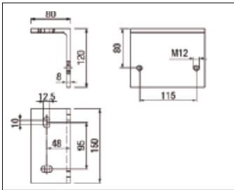
P333 Soporte de fijación para techo
