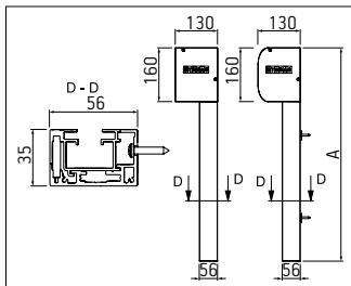
Montaje en fachada con soportes A = Altura total
