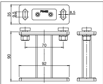
PS452/1 Soporte
