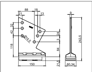
S725 Soportes para vigas
