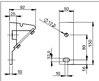
S831/5 Soporte para viga (desde el frente)
