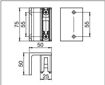
SR418 Conjunto de bisagras
