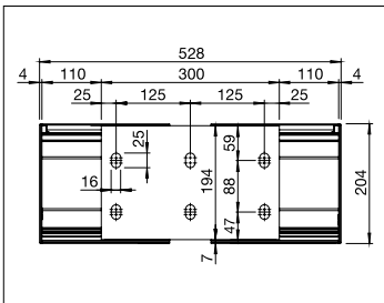
B423/2 Soporte de la guarnición 300 mm
