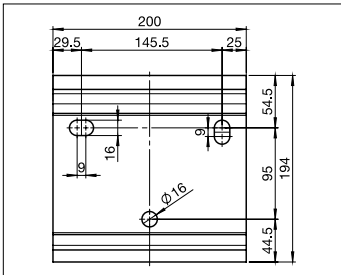
S563/1 Perfil de soporte L = 200
