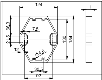
S821/1.. Distancia placas
