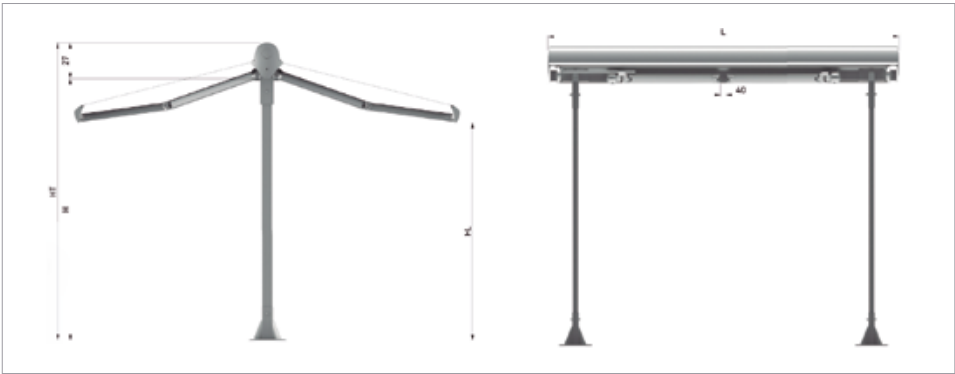
Dimensiones del sistema
