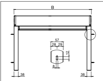
Dibujo de la instalación: al techo mediante montaje directo B = Anchura total
