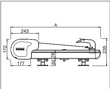
Instalación sobre estructura A = Proyección / salida
