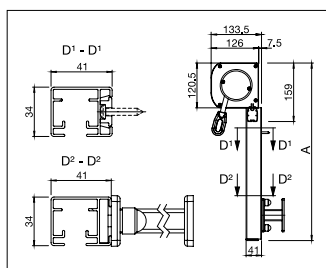
VS5200/1: Instalación a pared con clips A = Altura total
