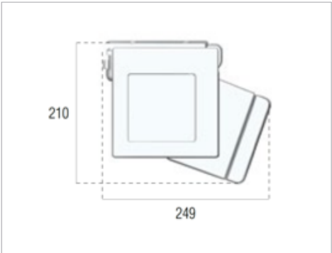
Instalación frontal
