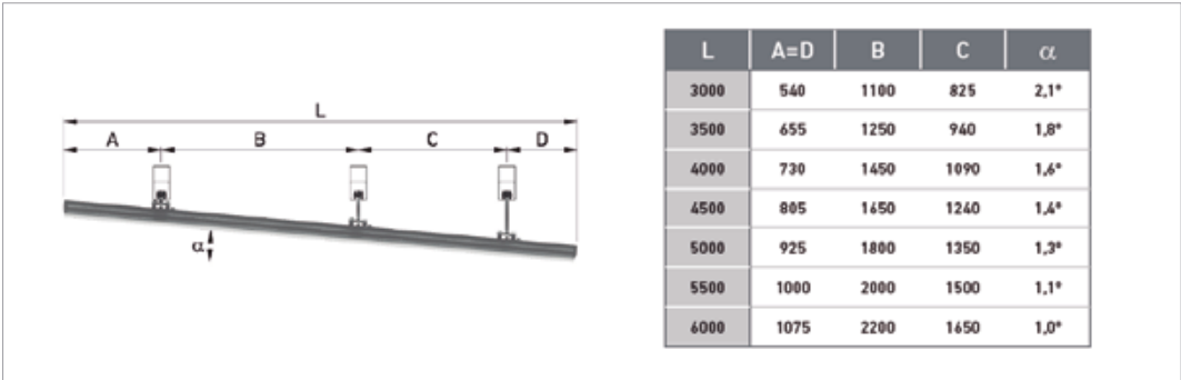
Dimensiones para pendiente
