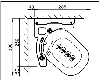
Instalación a techo 40°
