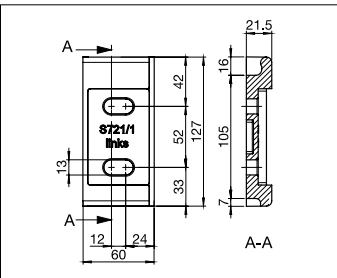
S721/1 Soporte
