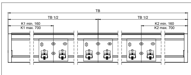
Plano de montaje (montaje a muro)
