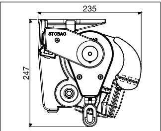
S8130 Instalación a techo
