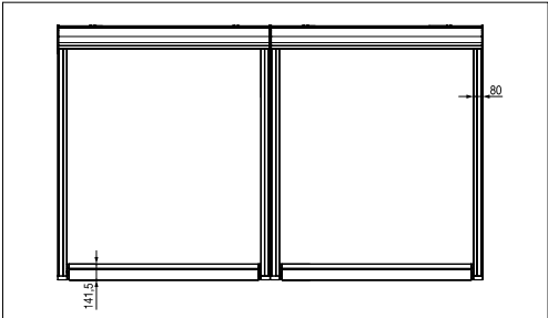
Vista superior de sistema con 3 guías
