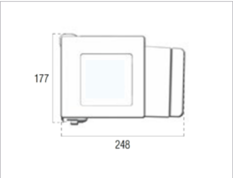
Instalación a techo
