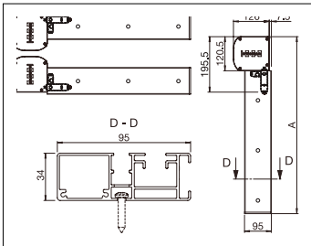
Instalación sofito A = Altura total
