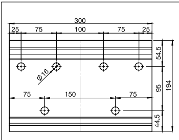
S563/2 Perfil de soporte L = 300
