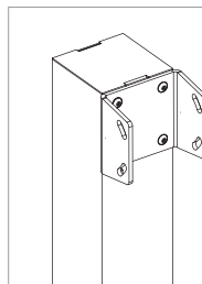
Soporte exterior para guía y perfil 100x120
