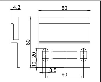
SR606 Instalación a pared
