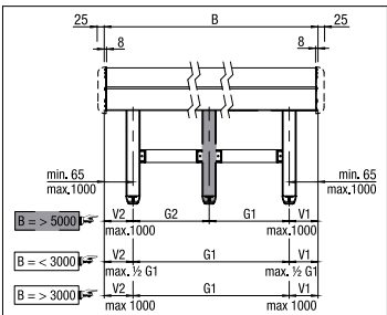
B = Línea total (sin PS619/.)
