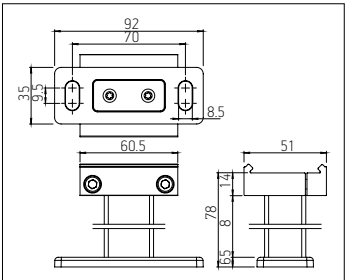
PS826-1 Soporte de fijación estándar (cajón pequeño)
