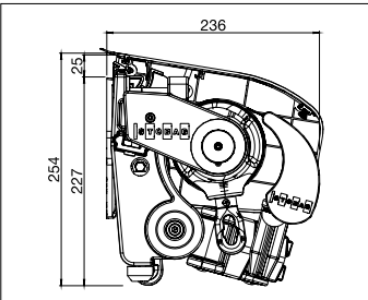
S8135 Instalación a muro
