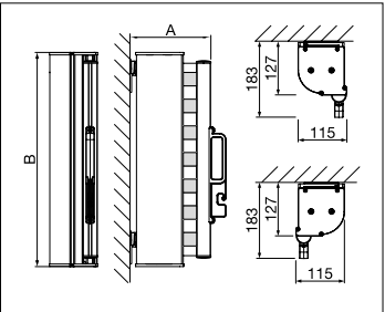
SR6000 Muro / Instalación superior
