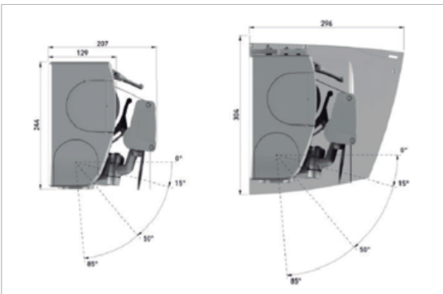
Dimensiones generales
