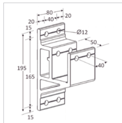
Detalle soporte (frontal y a techo)
