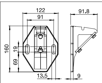
S831/3 Muro/Soportes para techo
