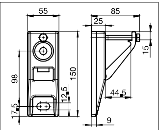
S821/2 Soportes pequeño techo/muro
