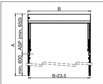
Plano de instalación W = anchura ASP = Punto al descubierto
