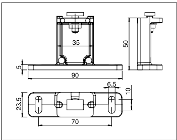
FS602/1 Soporte
