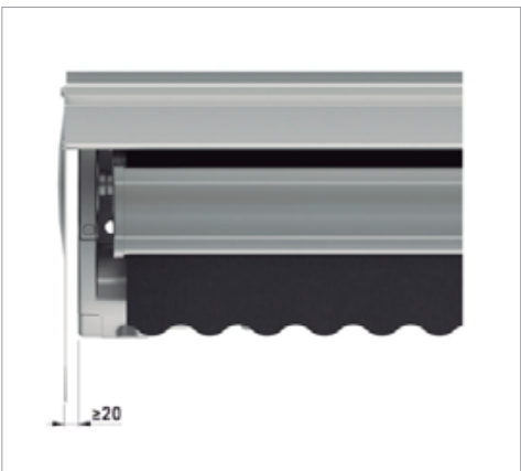
Distancia recomendada entre tapas y soporte
