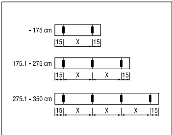
Posicionamiento y cantidad de soportes
