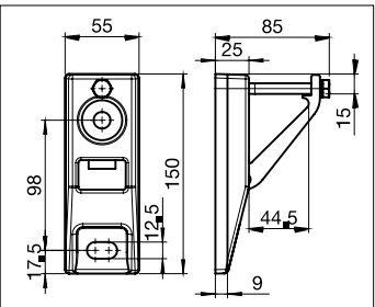
S821/2 Soportes pequeño techo/muro
