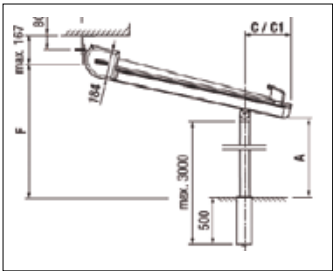
Montaje a muro con placa base
