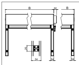
Disposición de los soportes con sistema de clips B = Ancho total
