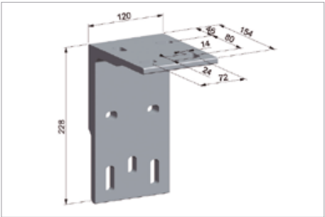
Fijación a techo ( + placa frontal)
