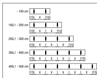
Configuración y número de abrazaderas de fijación / punzones o clips
