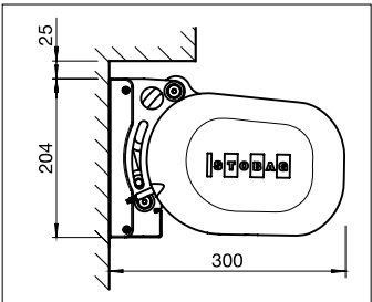
Instalación a pared
