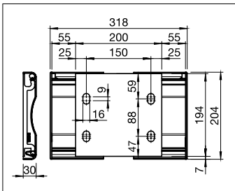
B423/1 Soporte de la guarnición 200 mm
