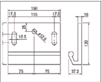
Soporte estándar
