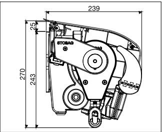
S8130 Instalación a pared con tejadillo S877/2
