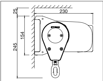
Instalación a pared Con rail frontal cuadrado
