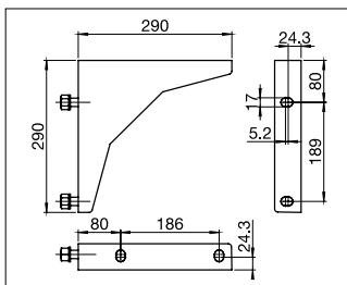
S346 Soportes para techo
