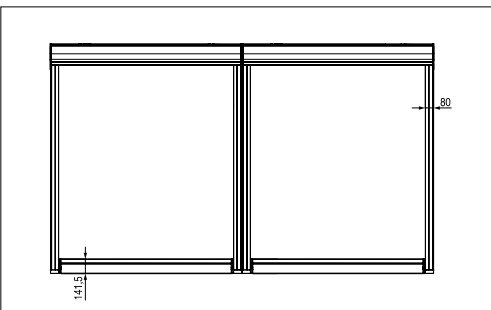
Vista superior de sistema con 3 guías
