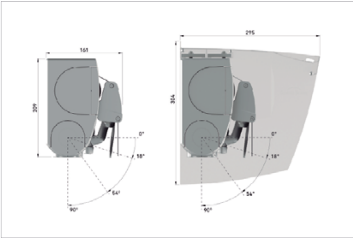
Dimensiones generales
