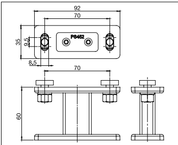
PS601/1 Soporte
