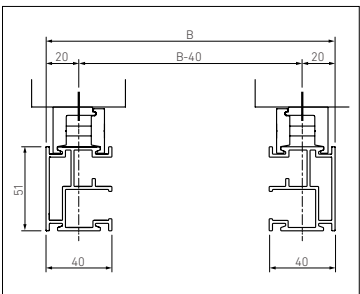
Vista de sección
