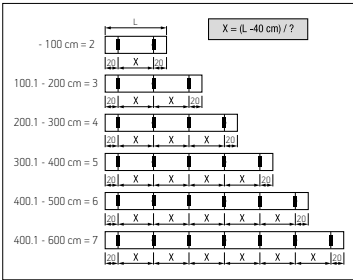
Reparto y nº de soportes con ZIP
