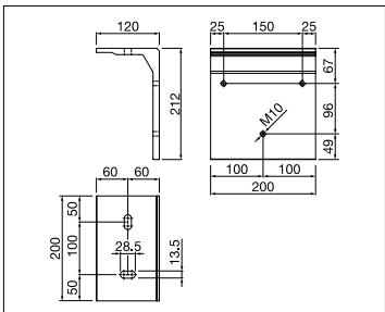
BX426 Herraje para montaje a techo
