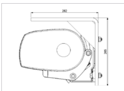
Fijación a techo - regulación mínima
