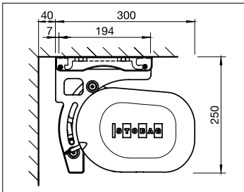
Instalación a techo
