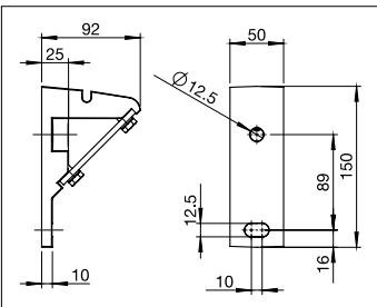
S831/5 Muro/Soportes pequeños para techo
