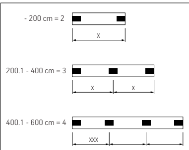
Reparto y nº de soportes (Cajón)
