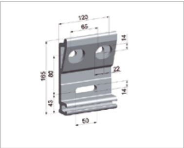
Placa para taco químico
