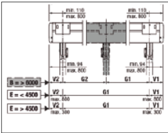
Plano de montaje B= Largo total
