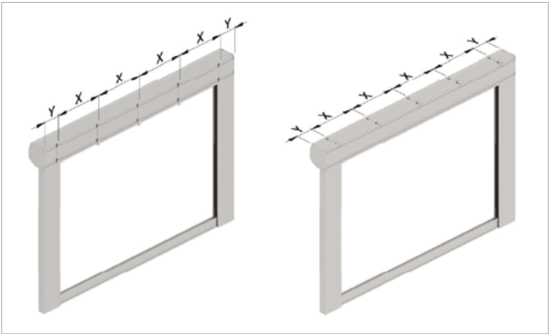
Distancia fijación a pared y a techo Y= 100mm X= 750mm
