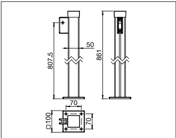
SR415/1 Kit poste para atornillar
