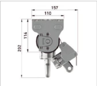
Dimensiones del sistema
