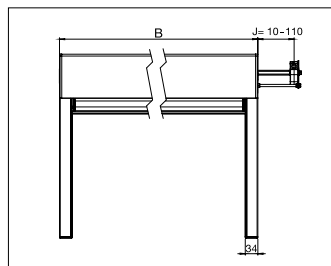
Disposición del soporte con el engranaje B = Ancho total
