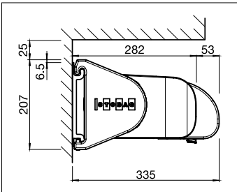
Fijación a pared con cenefa de caída Rail frontal redondeado
