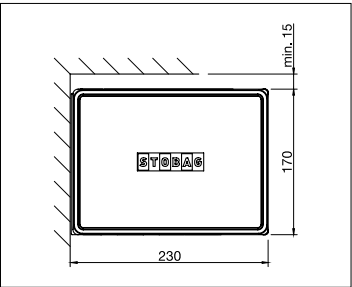
Montaje a muro
