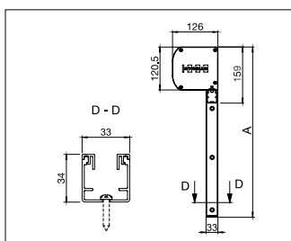
VS5200/2: Instalación a pared A = Altura total
