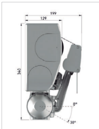
Dimensiones generales
