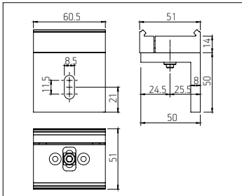
PS815 Soporte de fijación para techo
