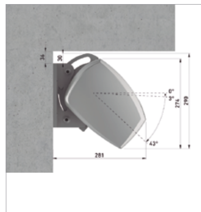
Detalle espacio necesario para instalación
