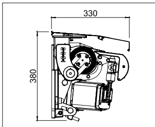
S247/3 Inst. a pared con tejadillo opcional
