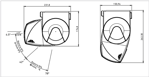
Fijación a techo
