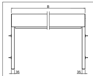
Disposición de los soportes, con motor B = Anchura total
