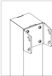
Soporte exterior para guía y perfil 100x120
