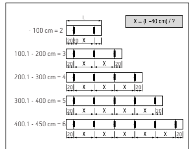
Reparto y nº de soportes (Rail guía)
