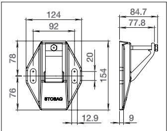
S821/1 Soporte techo/muro
