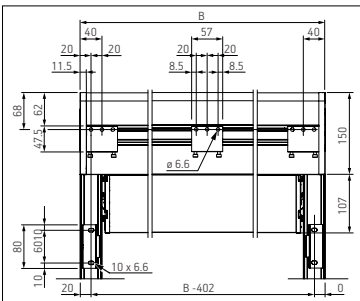
Plano de montaje B = largo total
