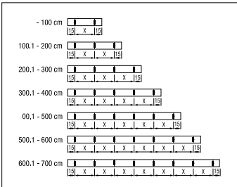
Configuración y número de abrazaderas de fijación
