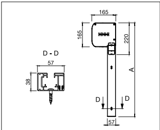
VS5600/2: Instalación a pared A = Altura total
