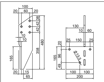
BX427 Soporte para vigas
