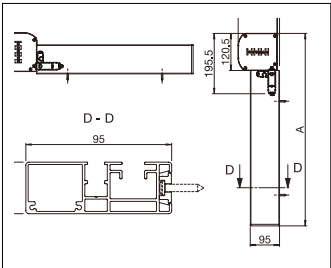
Instalación a pared con clips A = Altura total
