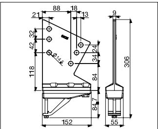
S825 Soporte para viga
