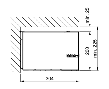
Montaje a muro
