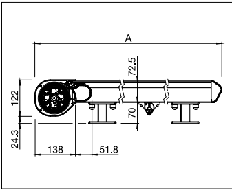
Instalación sobre estructura A = Proyección
