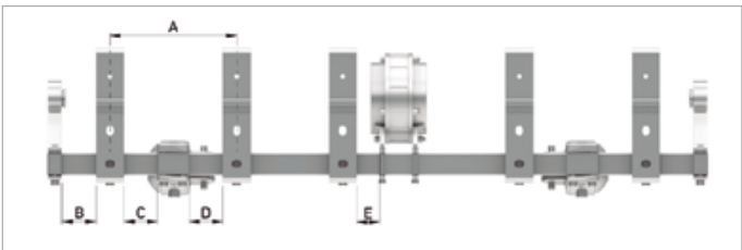
Fijación a muro
