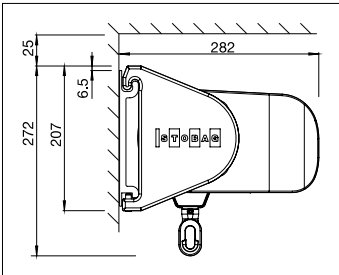
Vista lateral Instalación a pared - redondeado
