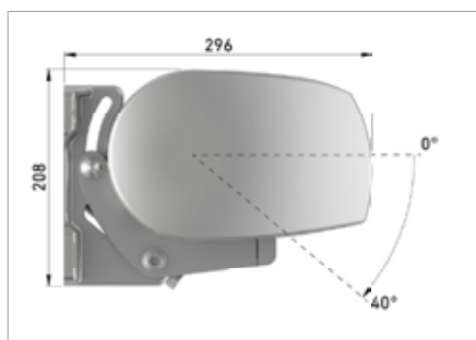
Fijación a muro - regulación mínima
