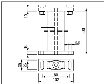
PS547 Soporte
